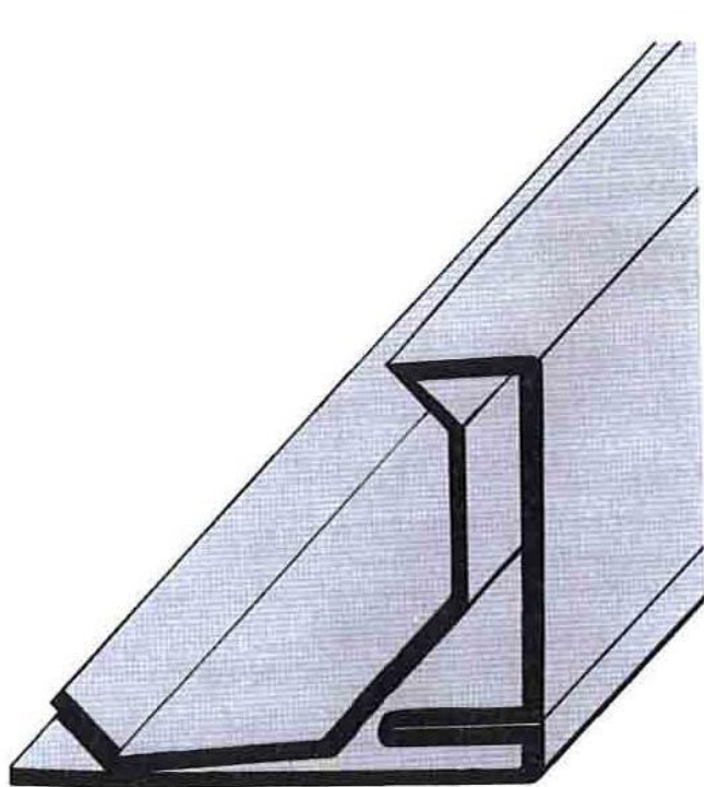
Профіль системи «S»
