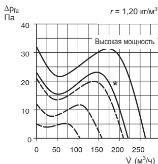
Диаграмма мощности M1/150
