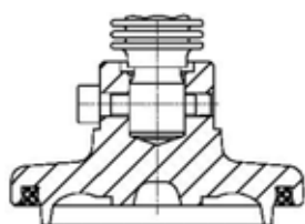
Дроссельная головка с уплотнительным кольцом из тефлона (PTFE), DN 15-100
