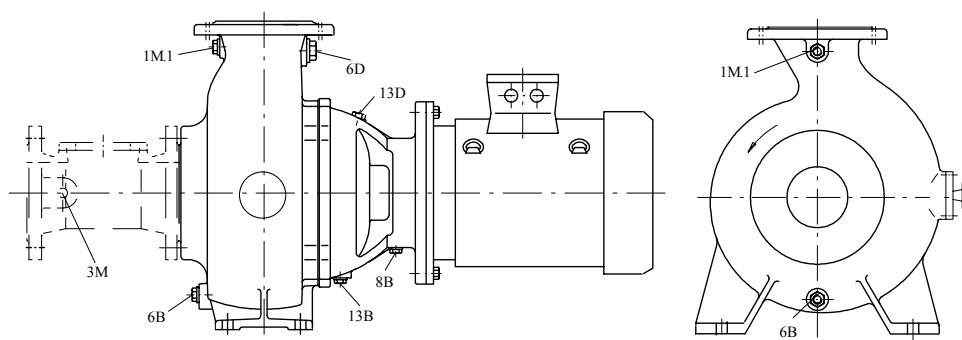
Рис. 6: Вспомогательные присоединения
