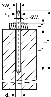
Рис. 4: Размеры
