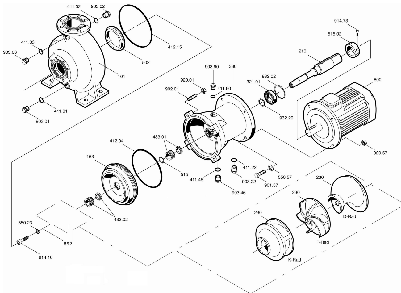
Рис. 17: Детализировочное изображение Sewabloc
