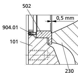
Рис. 14: Установка щелевого кольца
