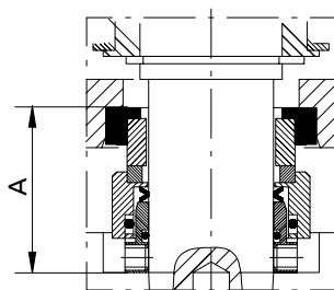
Рис. 13: Установочный размер «А»
