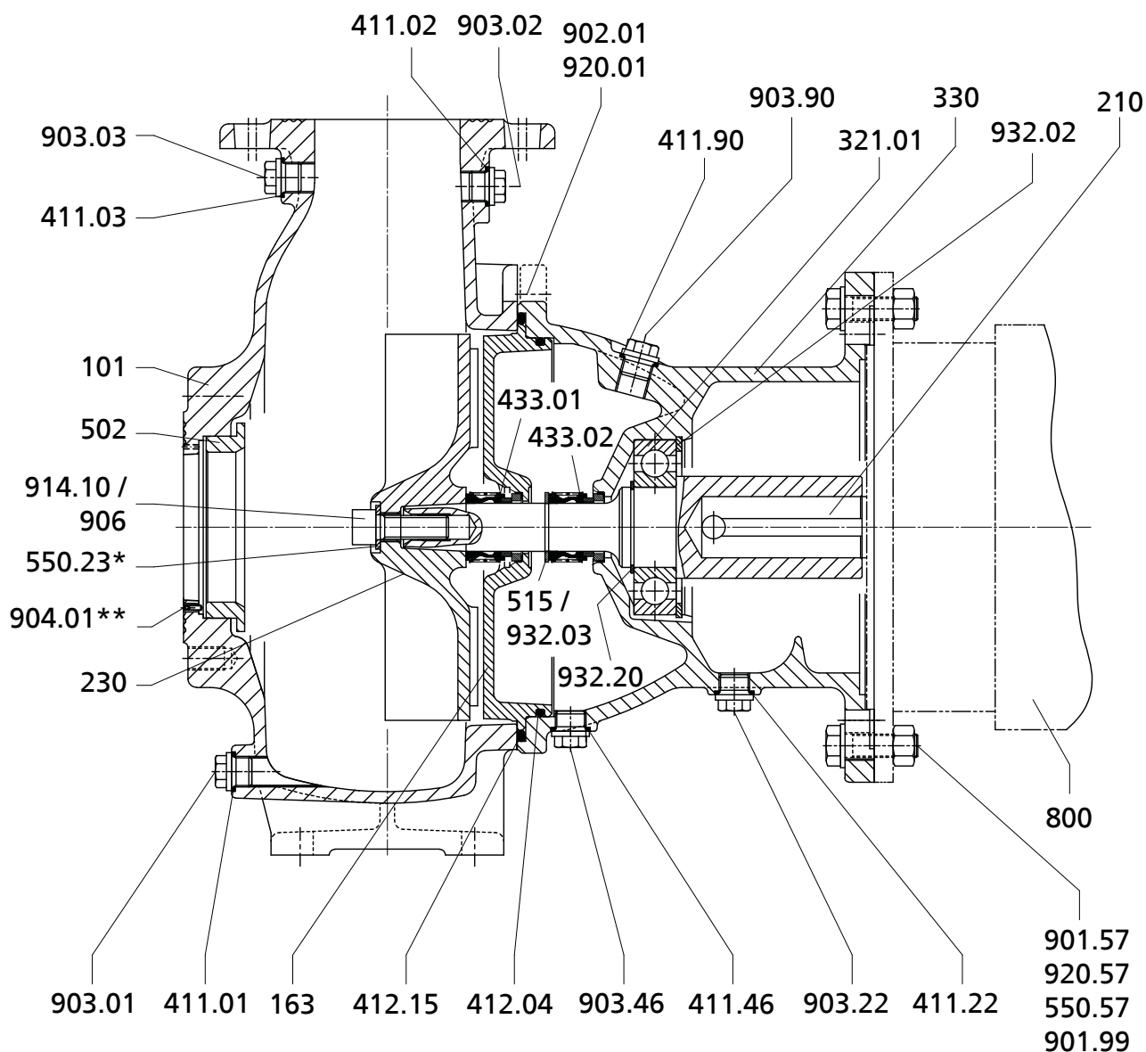
Рис. 16: Горизонтальная установка; * при наличии, ** только для типоразмеров 100-250, 100-251, 125-315, 150-315
