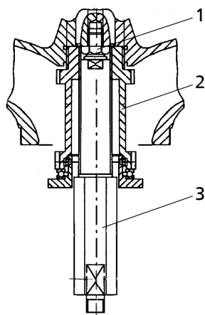
Рис. 20: Специальный съёмник
