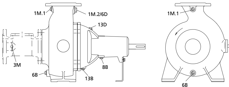
Рис. 6: Вспомогательные присоединения
