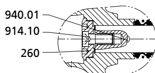
Рис. 19: Цилиндрическое соединения
