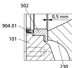
Рис. 28: Установка щелевого кольца
