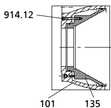
Рис. 23: Демонтаж износозащитной стенки
