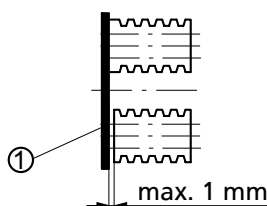
Рис. 8: Проверка ременного шкива
