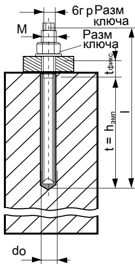
Рис. 4: Размеры
