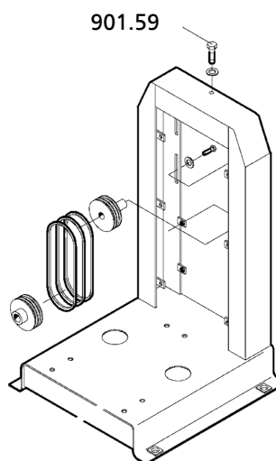
Рис. 9: Натяжение ремня
