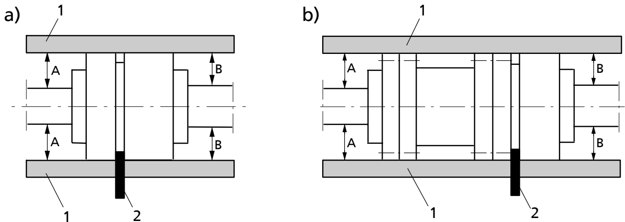
Рис. 7: Проверить центровку муфты: а) муфта, б) муфта с проставком
