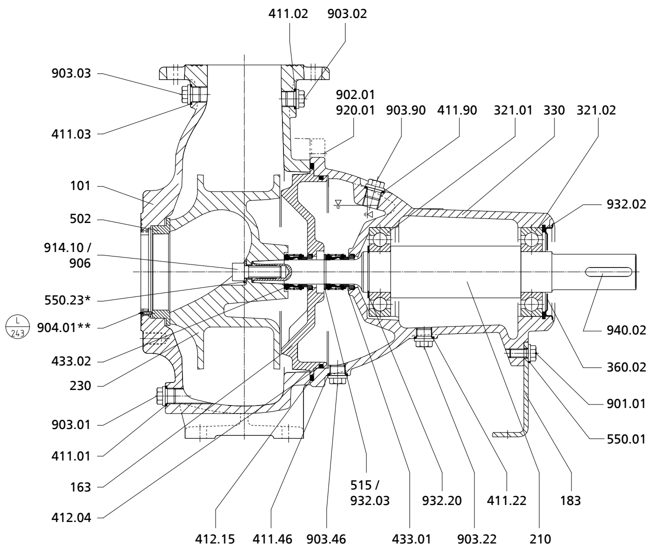
Рис. 30: Сечение с E-колесом
