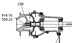
Рис. 18: Снятие рабочего колеса
