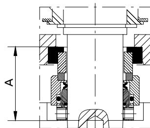
Рис. 26: Установочный размер "А"
