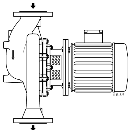
Рис. 9 Горизонтальная установка. Направление потока сверху вниз. Корпус насоса следует повернуть на 180° так, чтобы отверстия для отвода конденсата были направлены вниз, и клеммная коробка осталась в настоящем положении.
