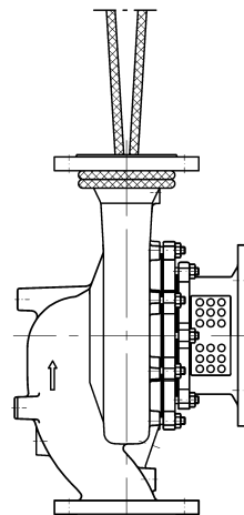
Рис. 2 Транспортировка насоса
